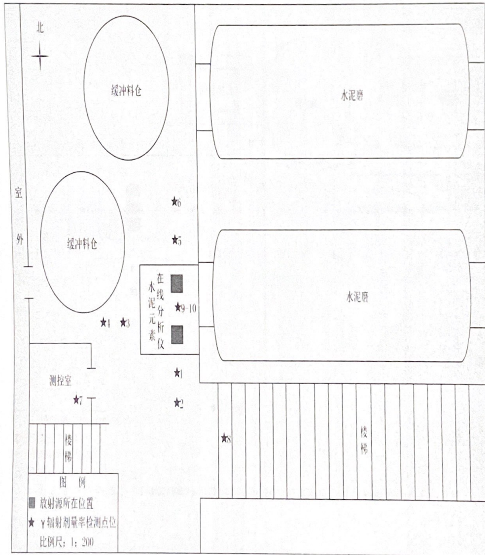
图 1 水泥元素在线分析仪 US15CF000684/US15CF000694 放射源监测布点示意图
